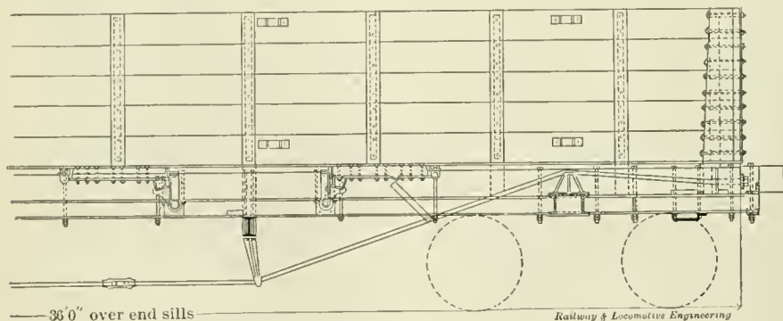
“SIX DOOR” GONDOLA—L. S. & M. S. Ry
